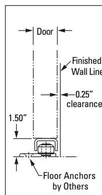
Bottom Door Guide
