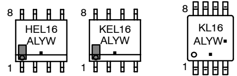
TSSOP-8
