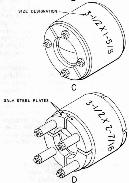
Fig. 3—Round Split Rubber Conduit Plugs
