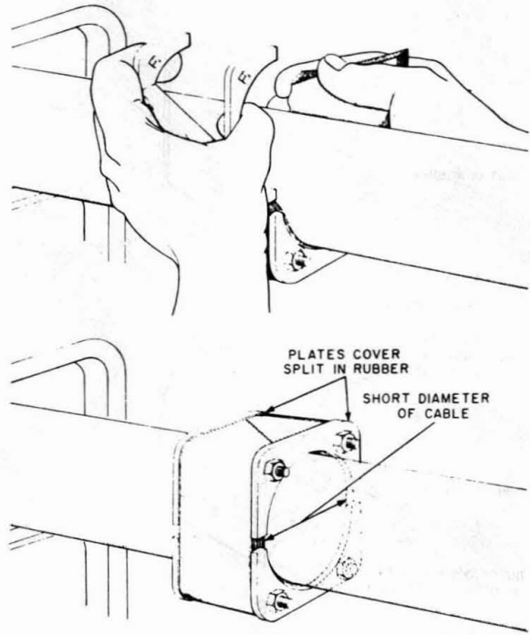
Fig. 4—Placing Split Rubber Conduit Plug on Cable
