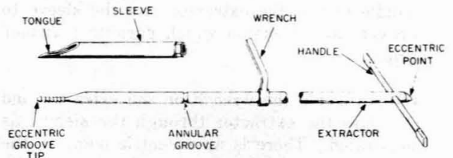
Fig. 6—Split Conduit Plug Remover
