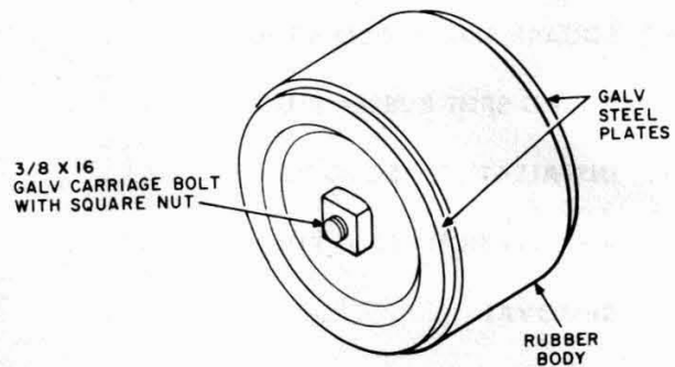
Fig. 1—Solid Rubber Conduit Plugs
