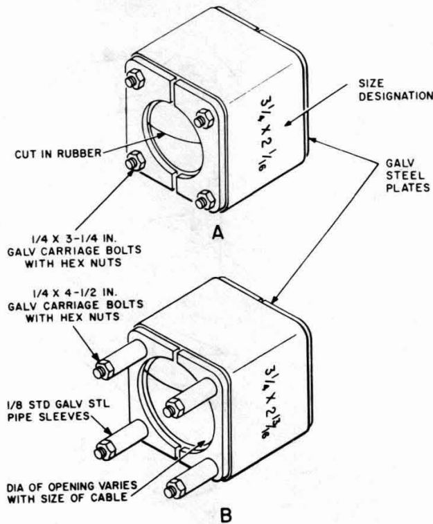
Fig. 2—Square Split Rubber Conduit Plugs
